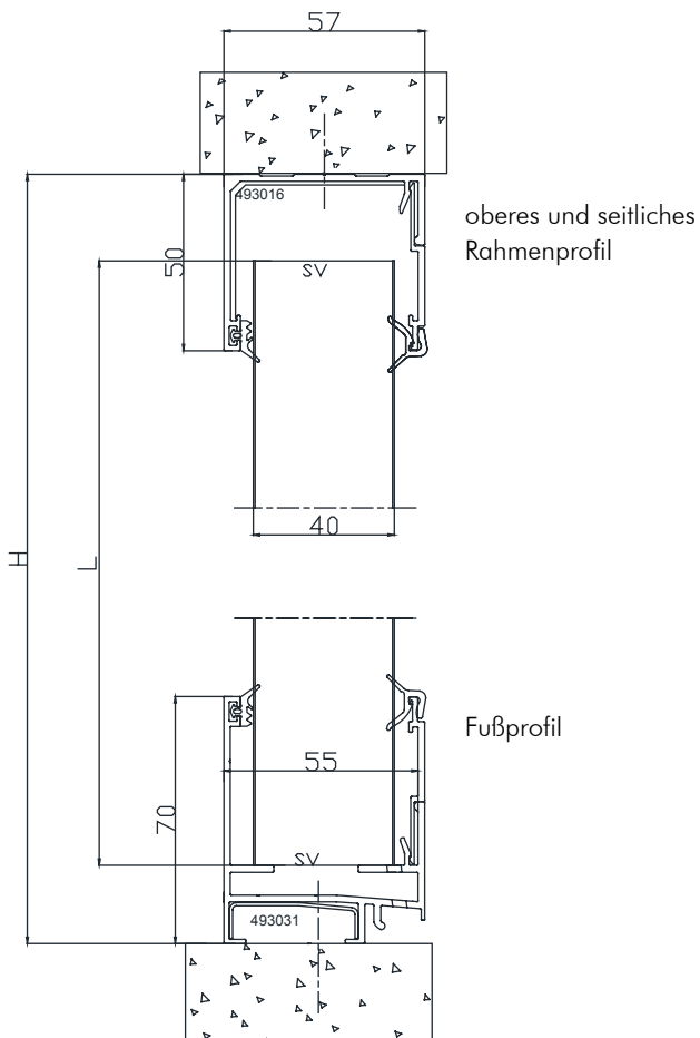
Beispiel 2 Montage in der Laibung z.B. bei Systemlängen bis 6 m
