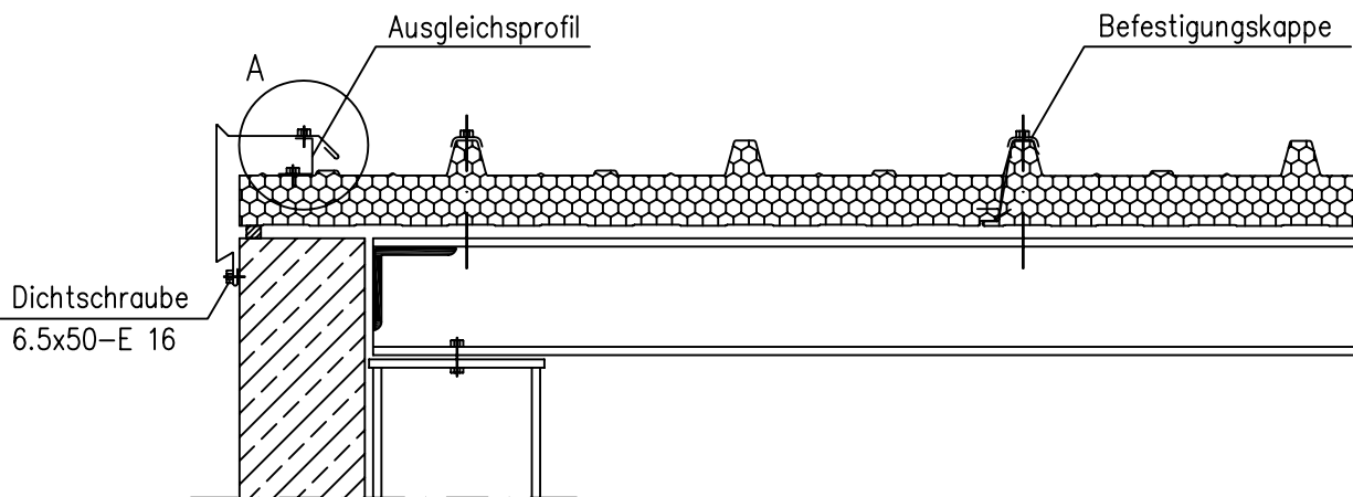
VERTIKAL-SCHNITT
