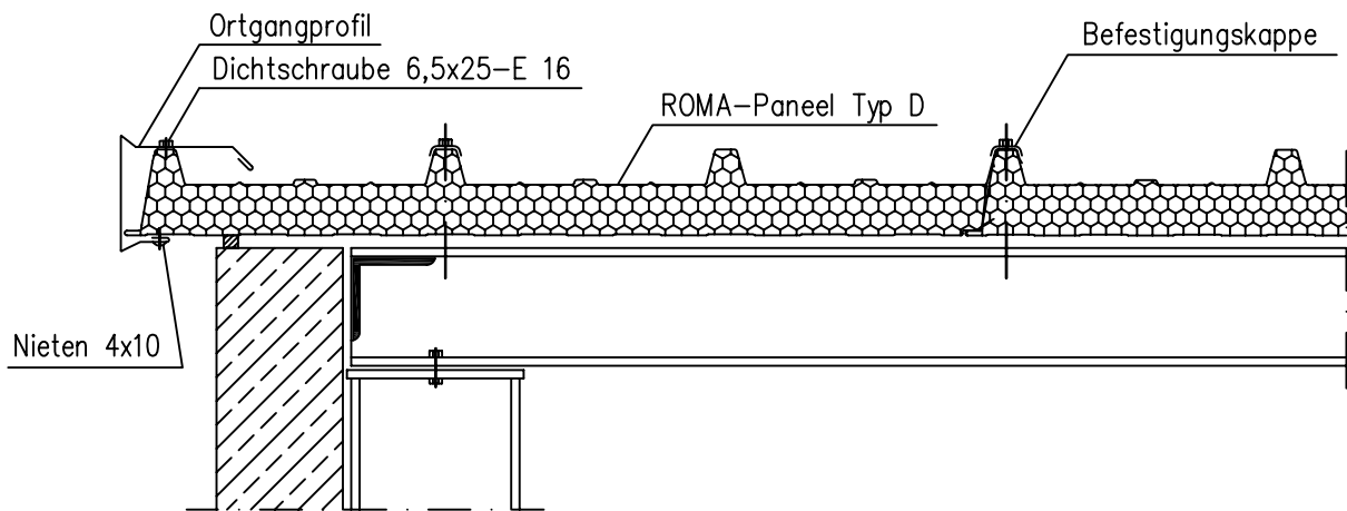
VERTIKAL-SCHNITT
