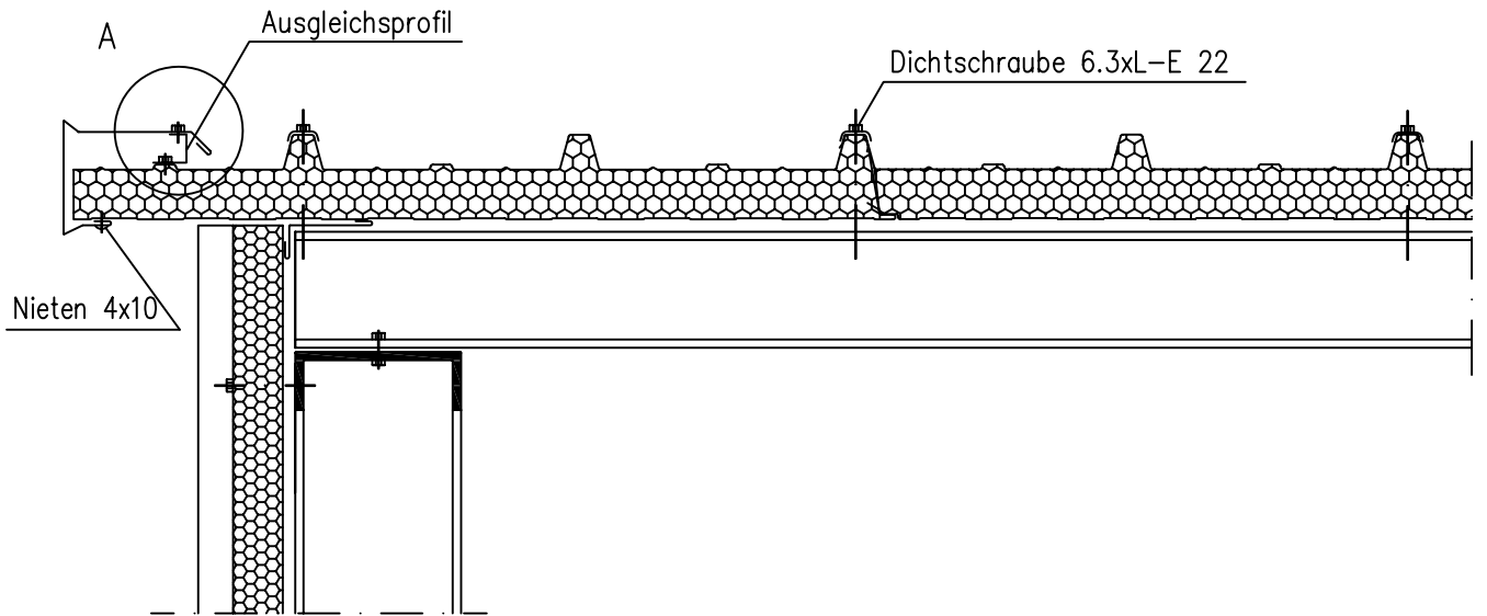
VERTIKAL-SCHNITT
